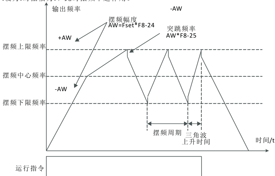
图5-24 摆频工作示意图
