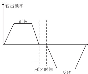
图5-02 正反转死区时间示意图
