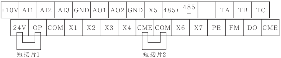
控制回路端子示意图
