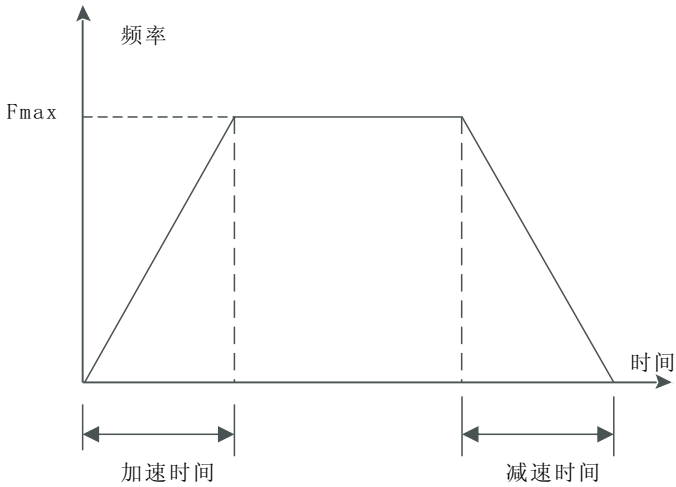
图5-20直线加减速
