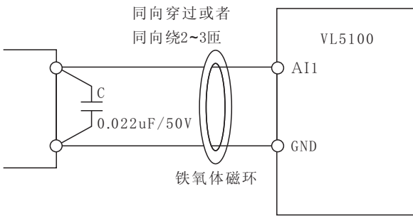
模拟量输入端子处理接线示意图
