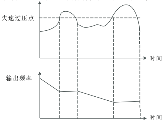
图5-26 过压失速功能
