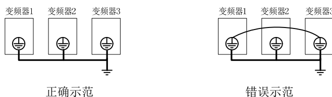
图 3-17 接地线接法示意图
