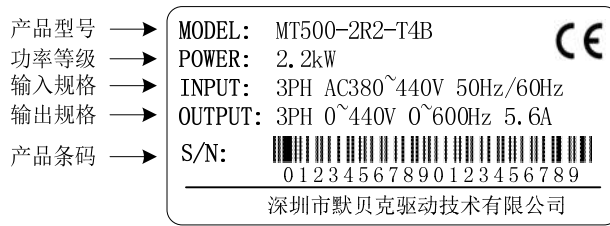
图 2-1 铭牌
