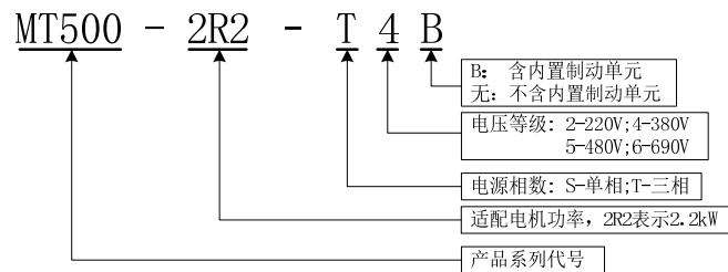
图 2-2 型号说明
