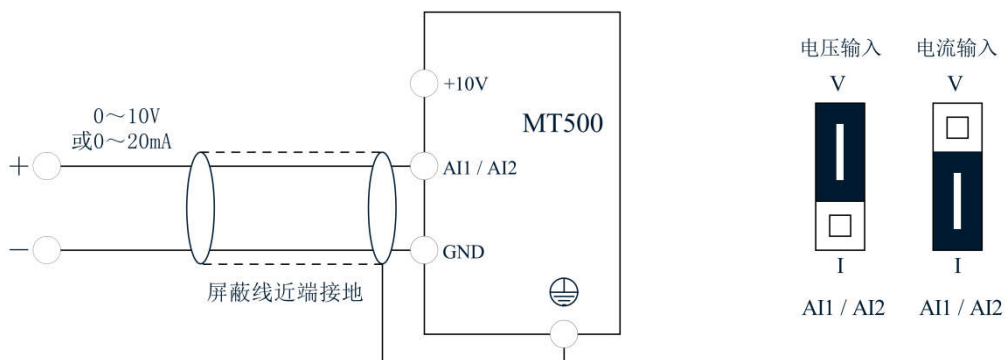
图 3-11 模拟量输入端子接线图
