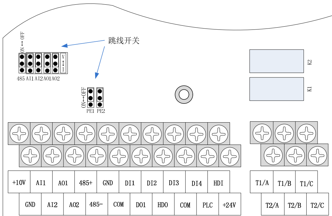
图 3-10 MT500 控制回路端子示意图
