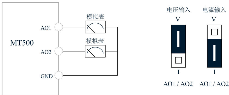
图 3-12 模拟量输出端子接线图
