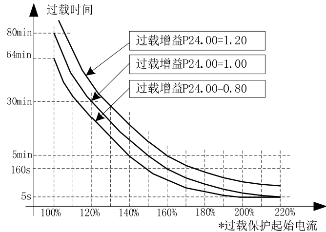
右图：不同过载保护增益下的电机过载保护曲线
