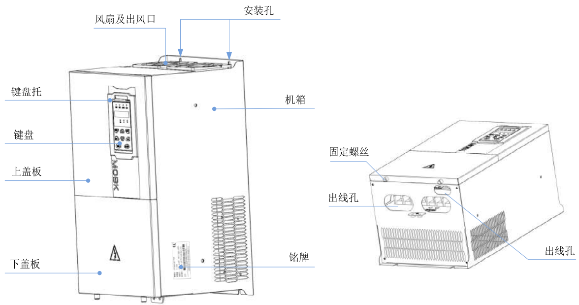
图 2-4 MT500 变频器 SIZE D~G 部件说明
