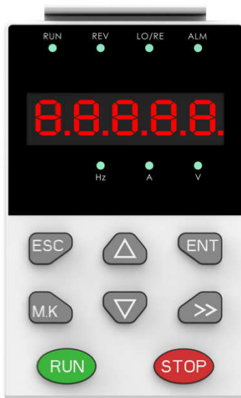
图 4-1 数码键盘
