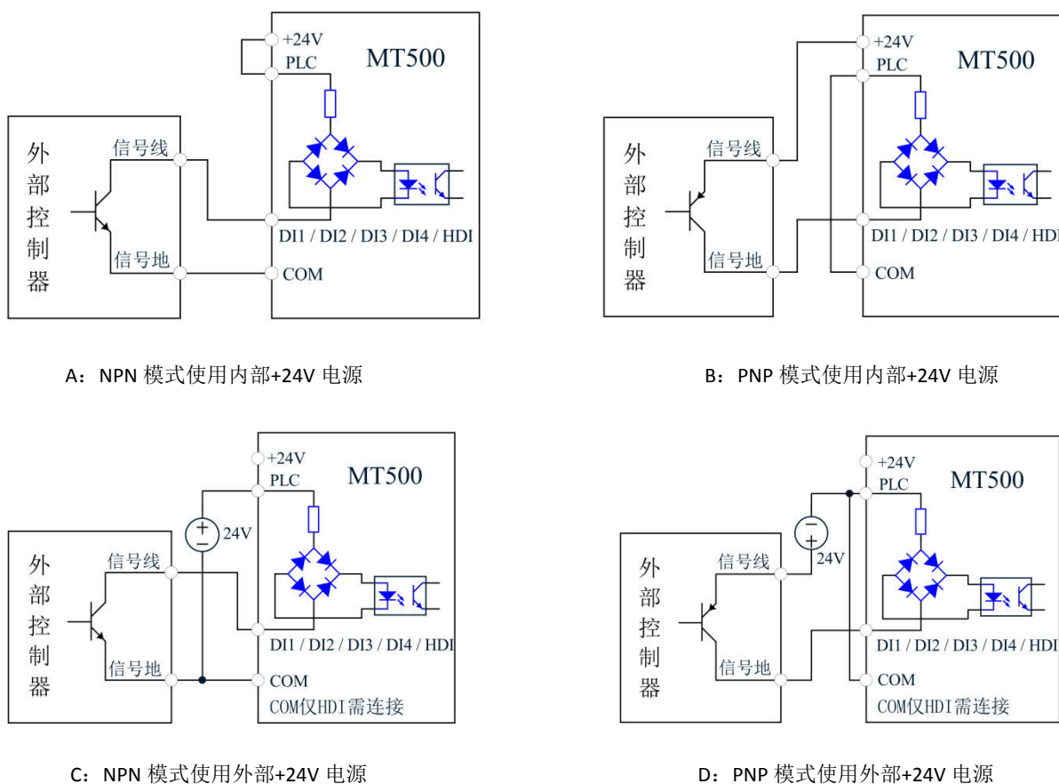
图 3-13 开关量输入端子接线图
