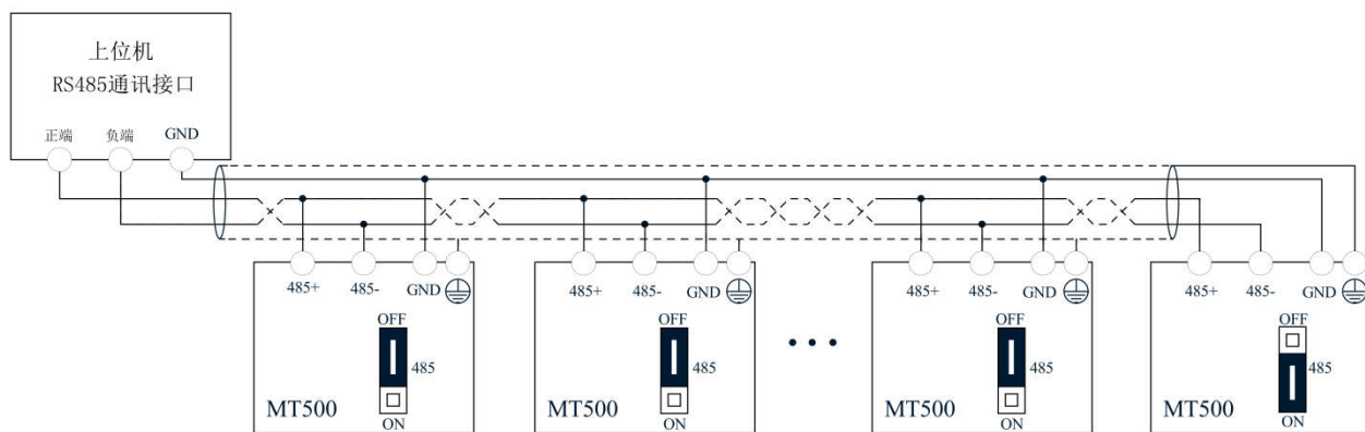
图 3-16 多台变频器 RS485 与上位机连接通信
