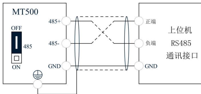
图 3-15 单台变频器 RS485 直接与上位机连接通信
