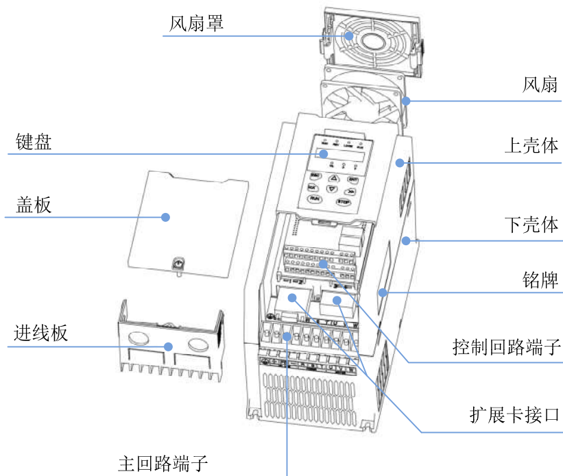
图 2-3 MT500 变频器 SIZE A~C 部件说明
