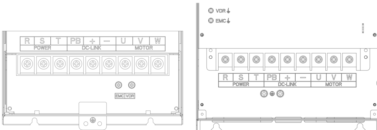
图 3-9 SIZE E (左)、F~G (右) 主回路接线端子示意图
