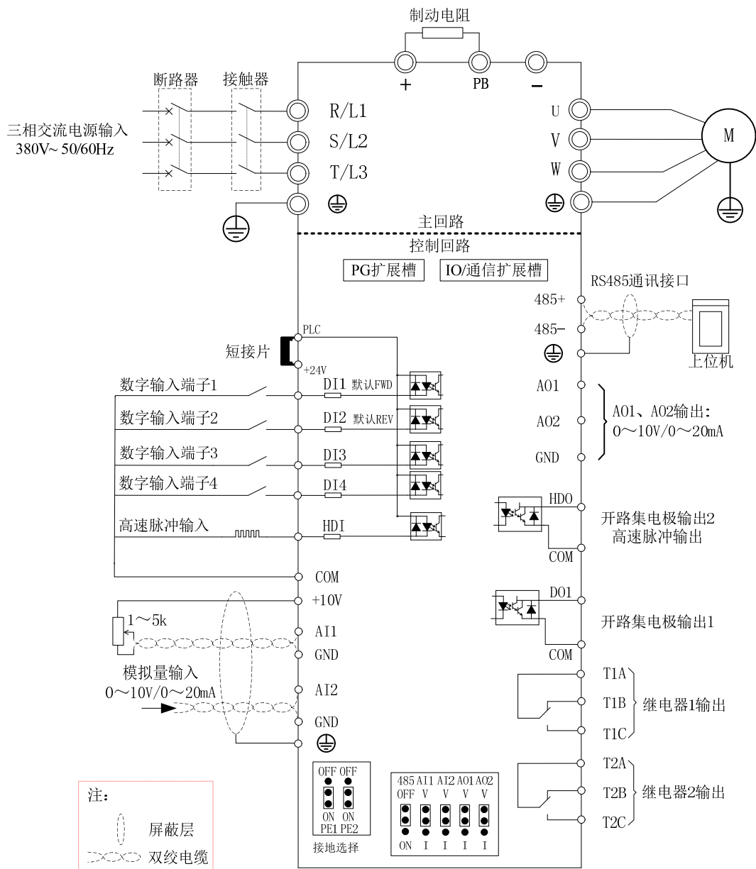
图 3-6 标准接线图
