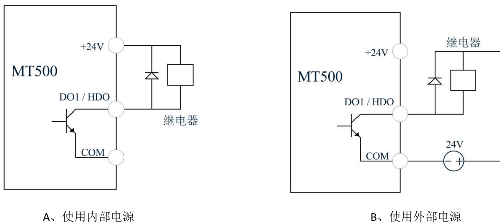
图 3-14 开关量输出端子接线图
